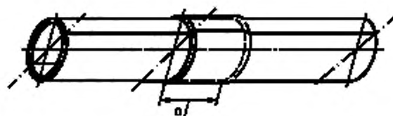
Рисунок D.3 — Контрольное соединение. Муфтовое нахлесточное соединение
